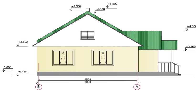
Ф А С А Д В О С Я Х Б - А Ф А С А Д В О С Я Х А - Б (зеркально)
